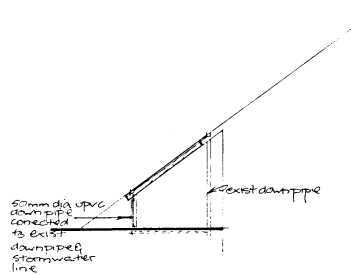
SIDE 1:100
